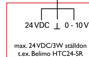
V2 Ställdon anslutning
