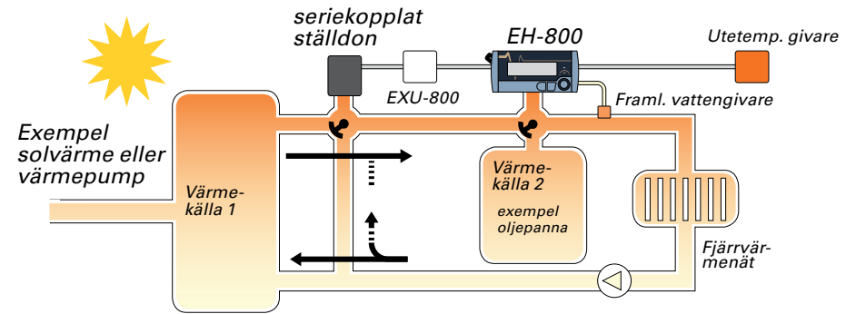
Bild ex. seriestyning. Inkoppling av seriestyrt ställdon.
